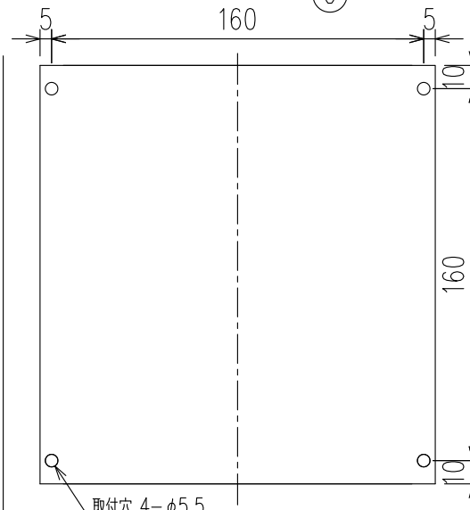
背面取付穴図
