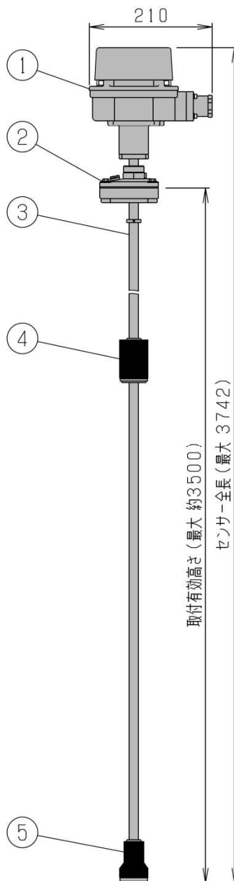
磁歪式液面センサー(デジタル容量表示機能付き) 《DSV-MSI-W》
