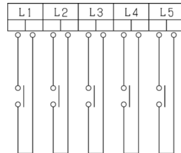
内部回路
