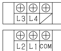
端子台配列
