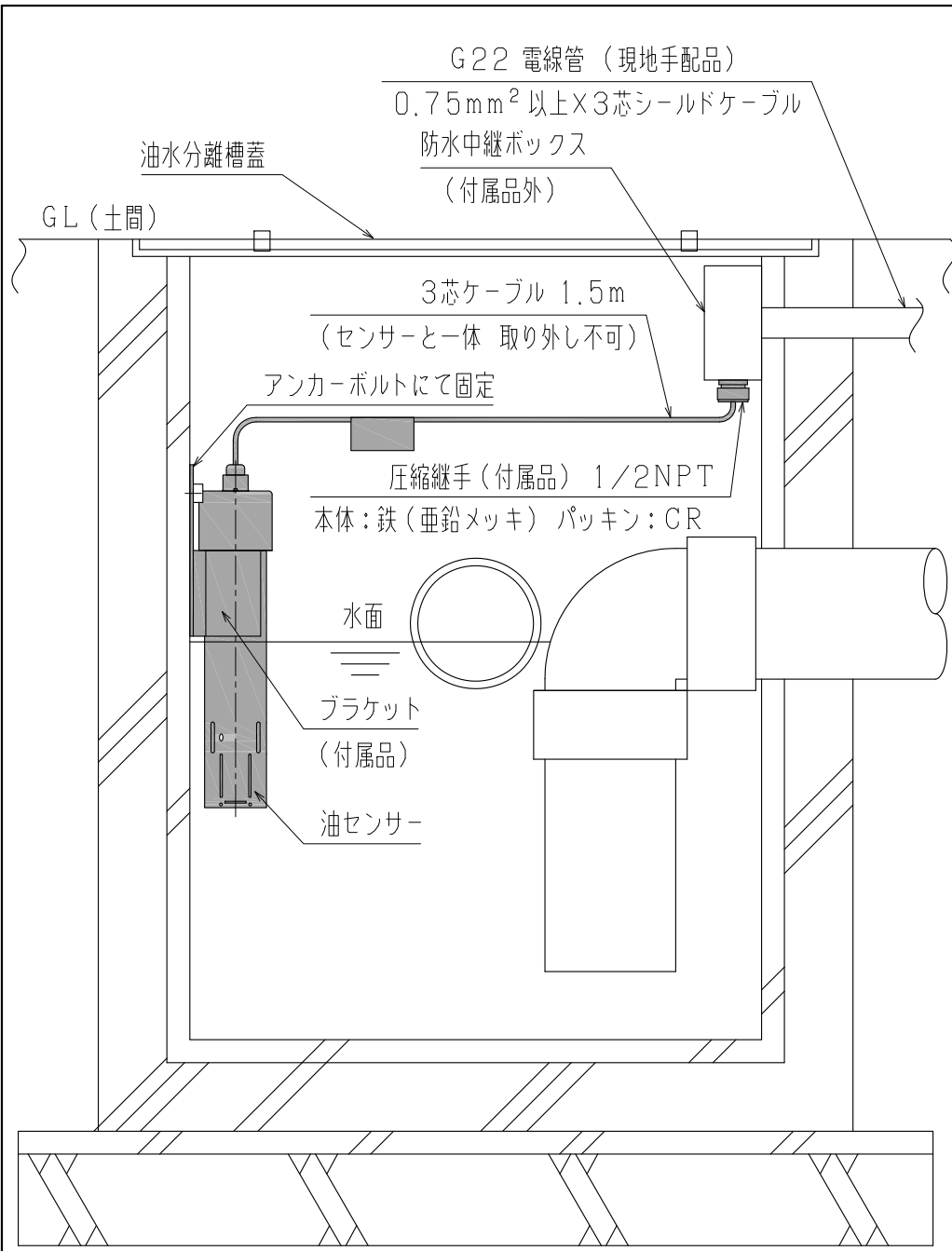
油水分離槽内設置図
